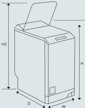
上置式洗衣機 Top Loading Washer
