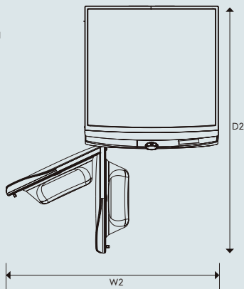
前置式洗衣機 Front Loading Washer
